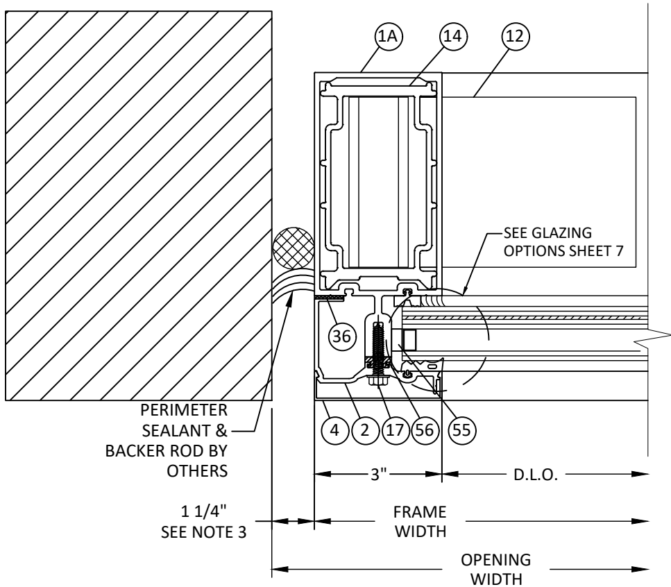
A 4 HORIZONTAL SECTION YHC 300 OG - JAMB
