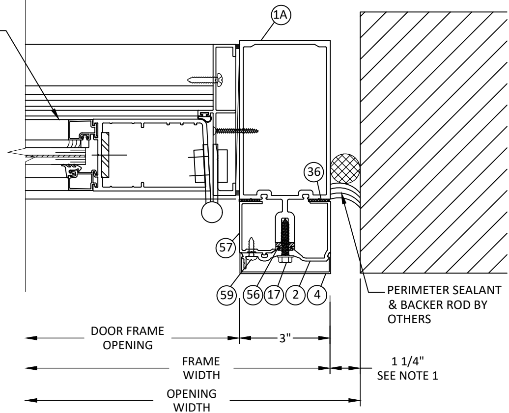
C 5 HORIZONTAL SECTION JAMB DOOR JAMB
